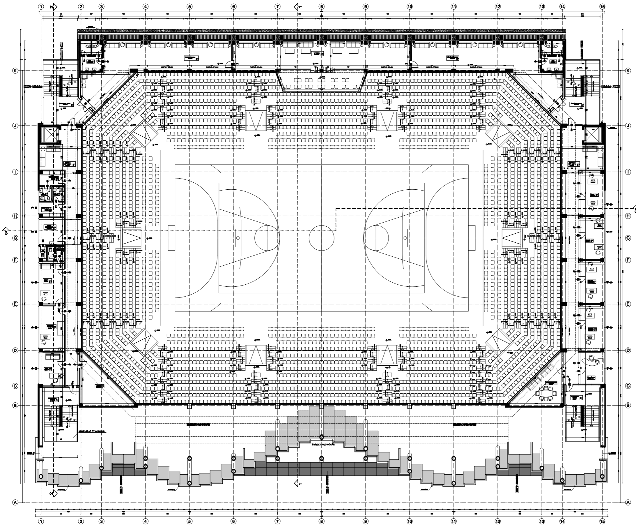
План II ниво М 1:200
