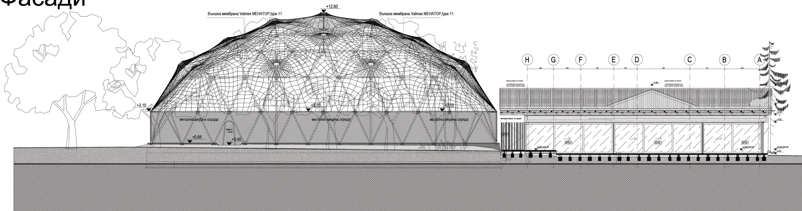
01 Фасада Изток
