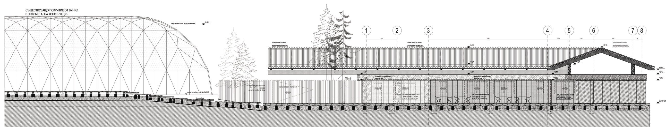
01 Фасада Юг
