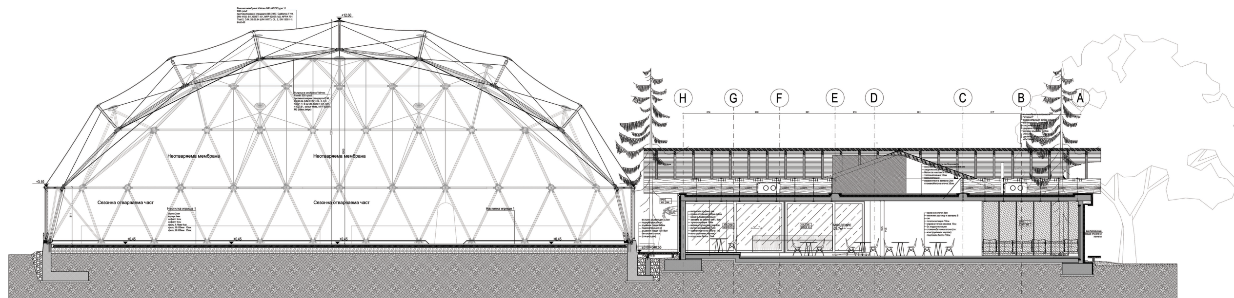
1-1 Разрез 1 - 1
