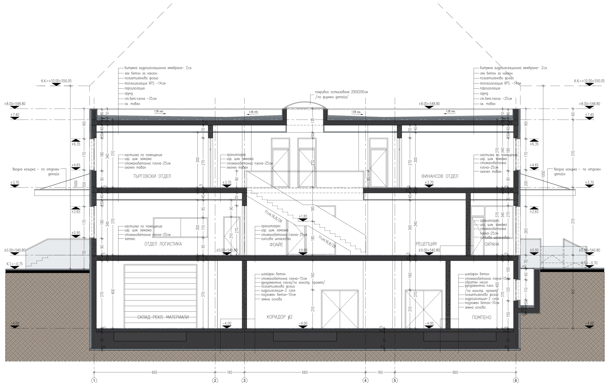
РАЗРЕЗ А-А
